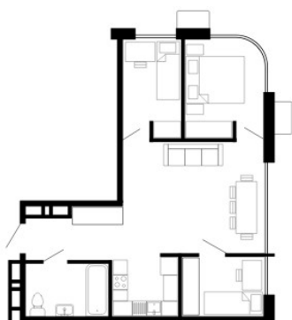
Планировка квартиры
